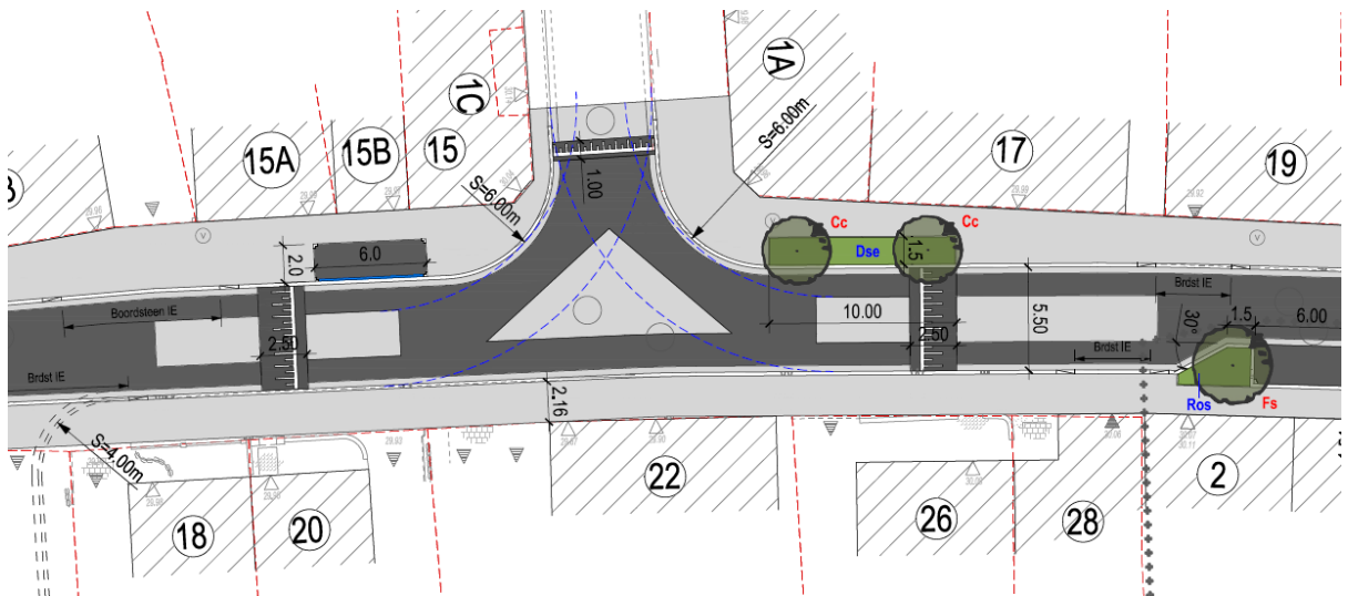
Figuur 1 : Verhoogd kruispunt Kapelstraat - Klokkenstraat
