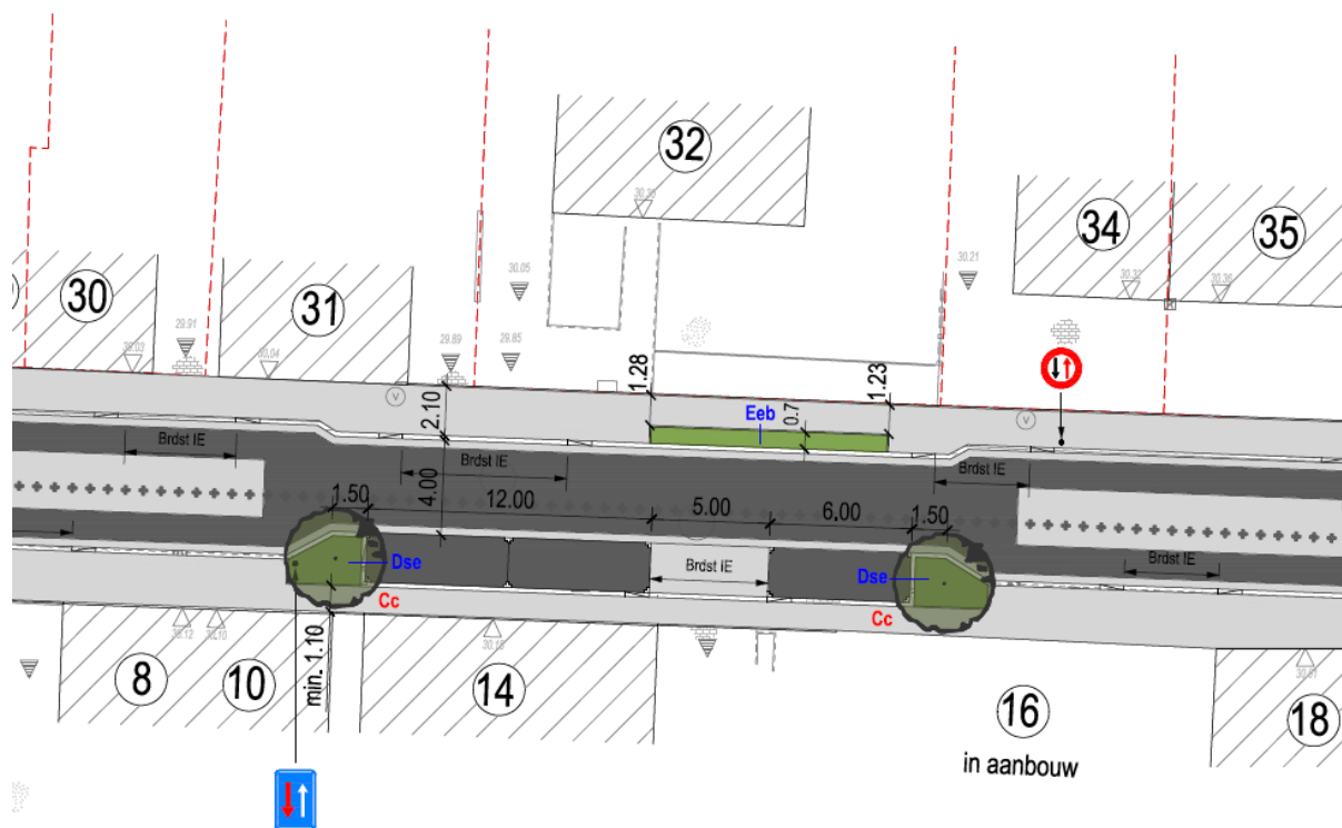
Figuur 2 : Wegversmalling thv nr 10 - 16
